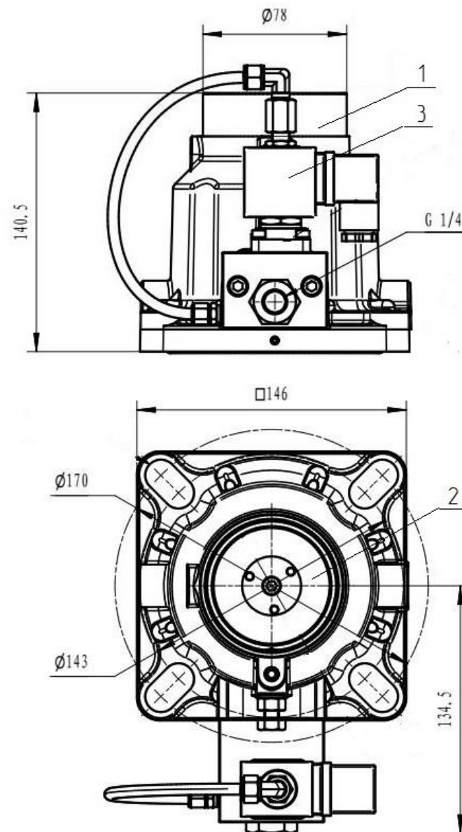
Рисунок 4. Клапан впускной.
