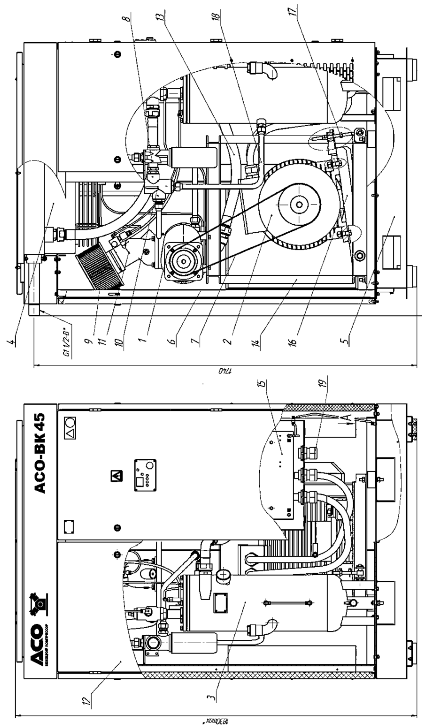
Рисунок 2. Установка компрессорная
