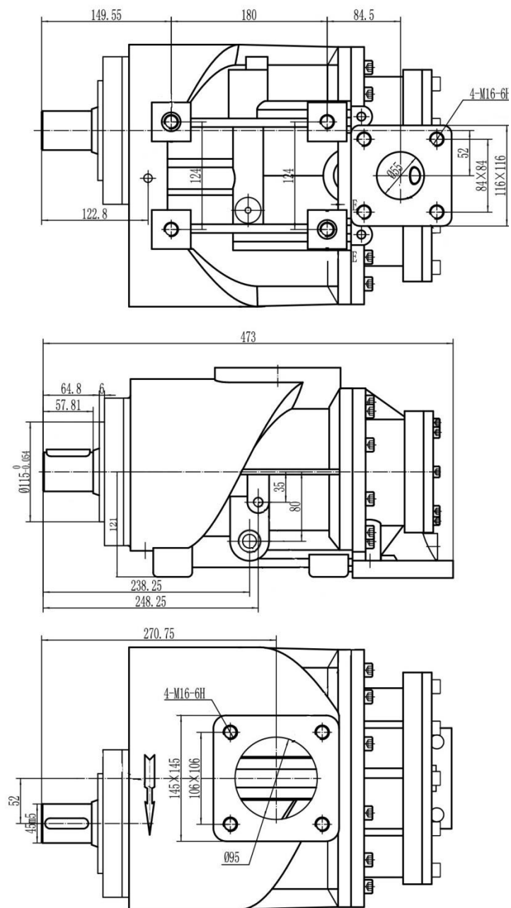
Рисунок 3. Винтовой блок.
