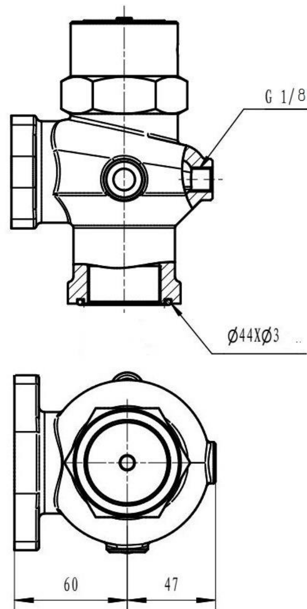
Рисунок 6. Клапан минимального давления.
